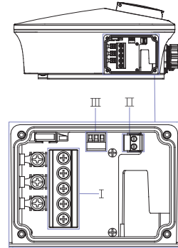
Three phase(11kW&22kW)
