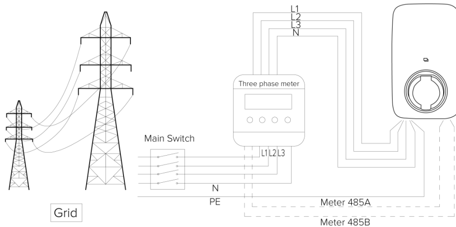
Three phase(11kW&22kW)
