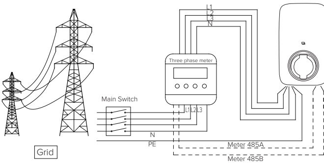
Three phase(11kW&22kW)
